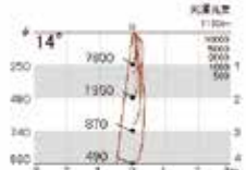
NPD-U100-15/30-NW[3000K]
