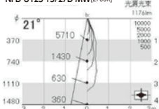
NPD-U125-15/27D-MW[2700K]
