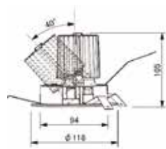
NPD-U100-15/30-NW[3000K]
